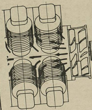
Luftkühlung, zwangsläufige Motorölkühlung
