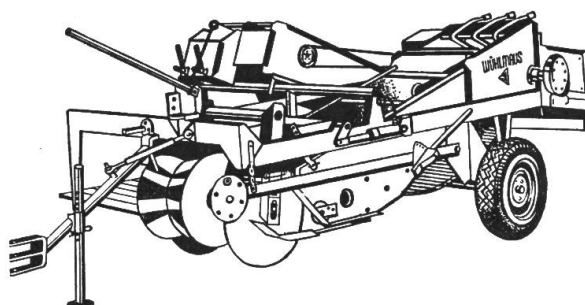
Sammelroder-Absackmaschine
