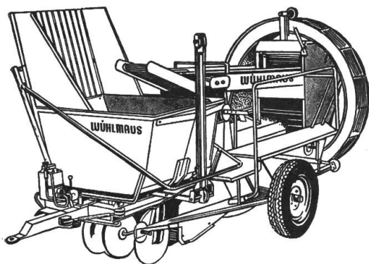
Vollernter-Bunkermaschine
