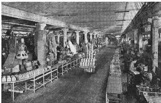
Teil-Innenansicht der SAME-Werke in Treviglio. Im Vordergrund sieht man mehrere Stück-Bearbeitungsmaschinen, von denen SAME die Mehrzahl selber entwickelt und gebaut hat.
