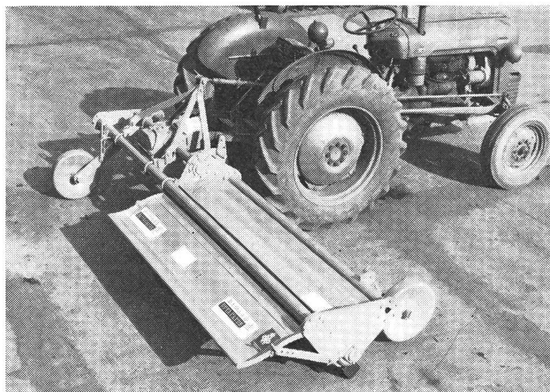
Abb. 2: «Howard» Seitenanbau- fräse. Der Fräskörper ist auf dem Rahmen verschiebbar.
