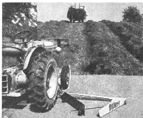
Mahdenformer an Traktoren Erbsheber und Abstreifer Maismähergerät «Kemaïs» (pat.)
