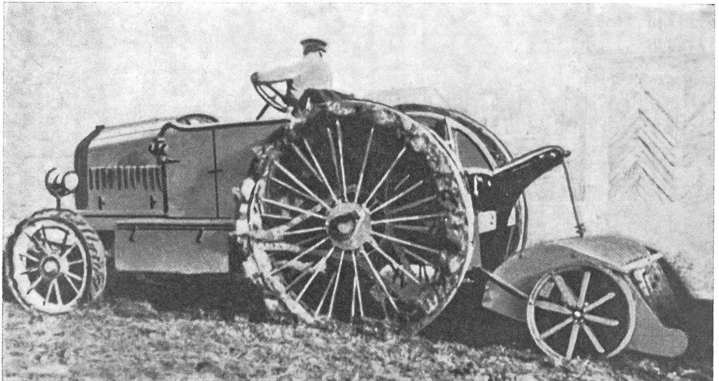
Traktor «Berna» mit Frässhwanz. Jahrgang 1918. Damals hergestellt von der Lastwagen- fabrik «Berna» in Olten.
