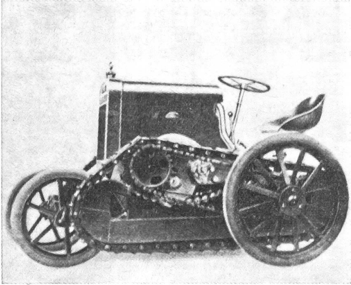
Kombinierter Rad- u. Raupentraktor. Jahrgang 1928. Hersteller: Süddeutsche Maschinenfabrik.
