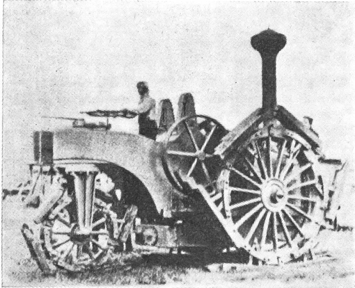
Englischer Dampftraktor aus dem Jahre 1875. Gewicht: 20 000 kg. Motor: 100 PS.
