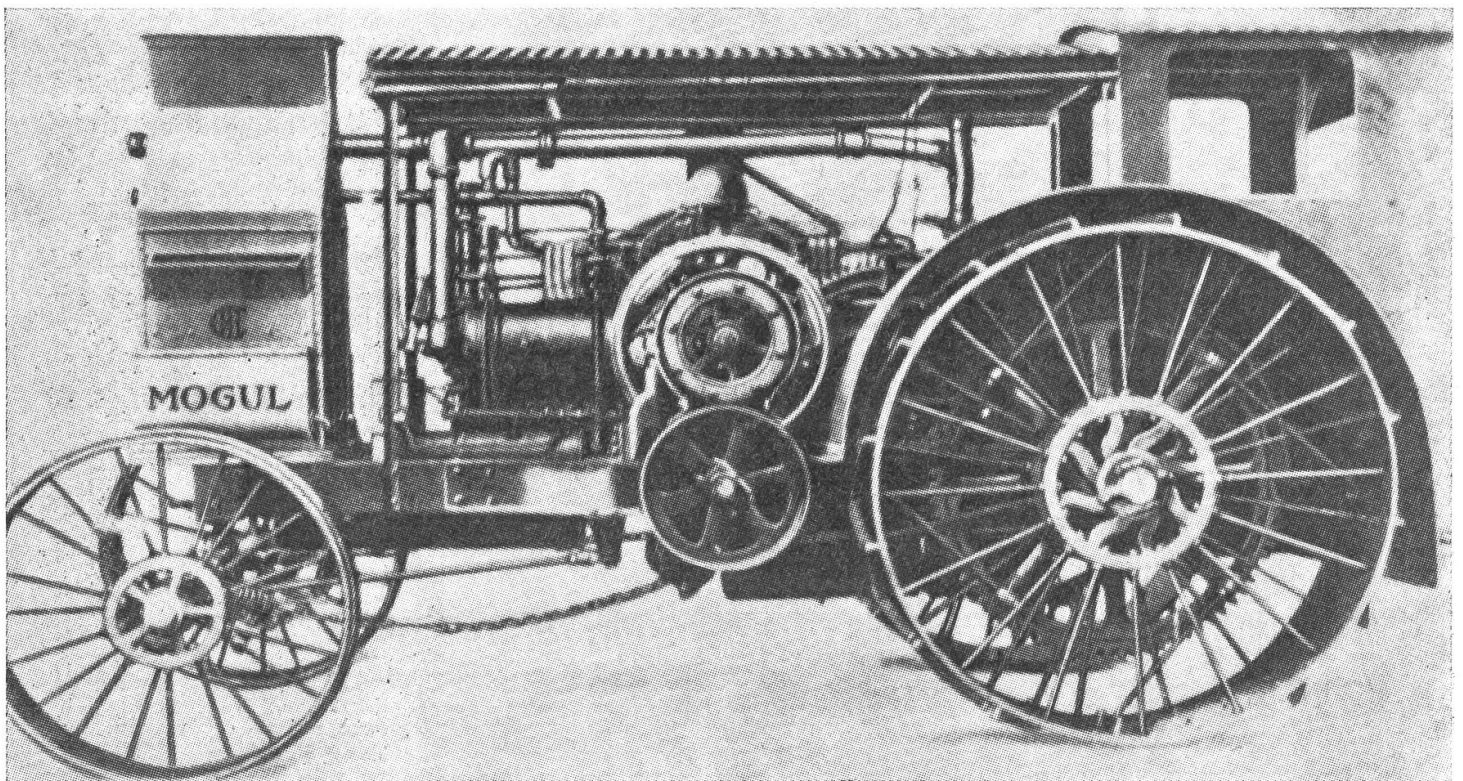
Amerikanischer Traktor «Mogul» (IHC). Jahrgang 1910. 45 PS. Gewicht: 11 Tonnen.
