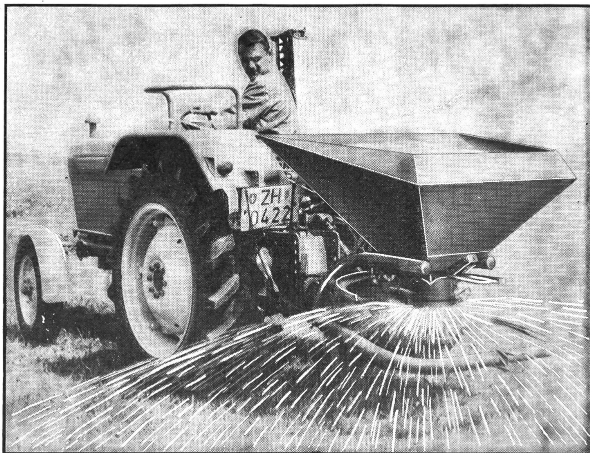
LELY-Düngerstreuer
