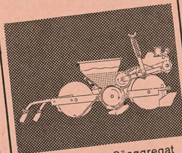
Schnitt durch ein Säaggregat der Einzelkorn-Sämaschine
