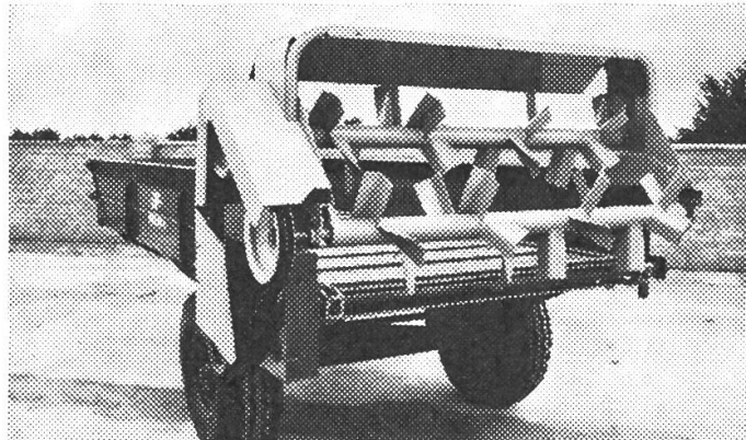
Der <JF>-ALLZWECKWAGEN als 5-Tonnen-Mistzetter mit dem neuen Doppelstreuwerk. Der ideale Miststreuer für Maschinengemeinschaften.
