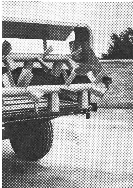
Streuzer mit dem neuen Doppelstreuwerk. Die Streuung erfolgt über die Zapfwelle.
