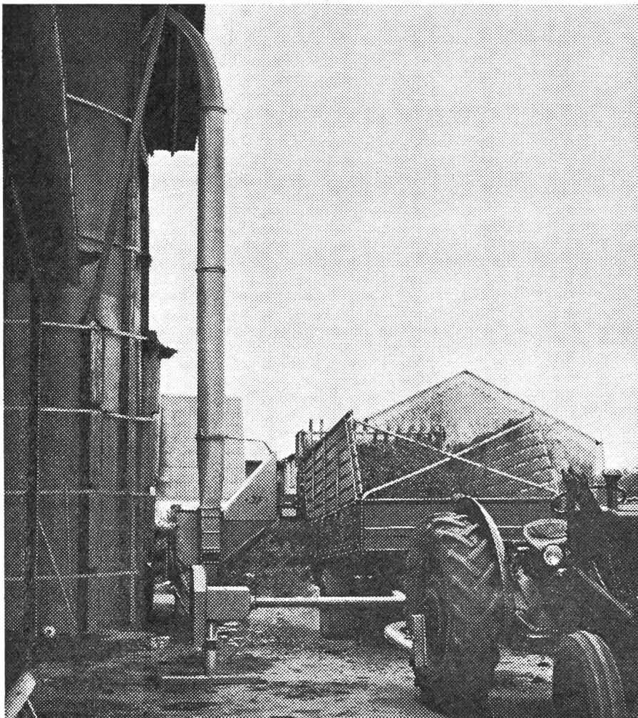
Das JF-SILOWURFGEBLÄSE (Zapfwellenantrieb) und der JF-Allzweckwagen (als Häckselwagen) mit dem Kombi- und Seitenabladner beim Füllen des Silo.
