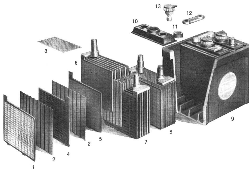
Abb. 1: Die Bestandteile einer Batterie:
