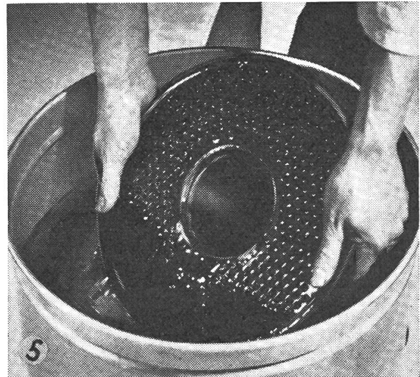
5 Filtereinsatz mit Dieseltreibstoff auswaschen
