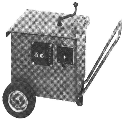
Standard, fahrbar N3/30—250 Amp. stufenlos 380 V, 65 kg Fr. 770.—
