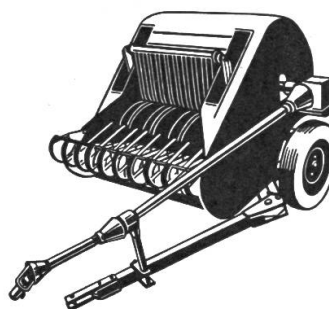
Niederdruck-Sammelpresse F 81 zum Pressen und Laden von Heu und Stroh. Aufnahmebreite 1,4 m Stundenleistung 4 bis 8 Tonnen Mit Grünfutterelevators lieferbar
