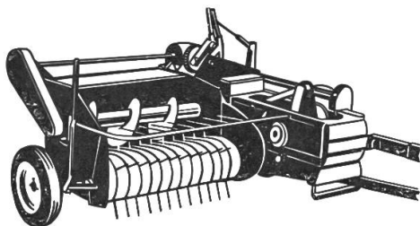
Hochdruck-Sammelpresse Typ 214 T + Typ CB 300 für Heu und Stroh Aufnahmebreite 1,60 m, Stundenleistungen: Stroh 7 Tonnen, Heu 9 Tonnen
