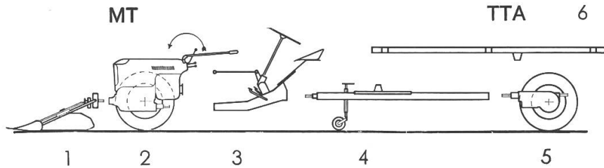
MT-TTA (2+3+4+5+6) = Gelände-Universal-Lasttraktor und Nutzfahrzeug mit Vierradantrieb.
