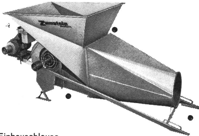
Einbauschleuse für Versenkgrube
