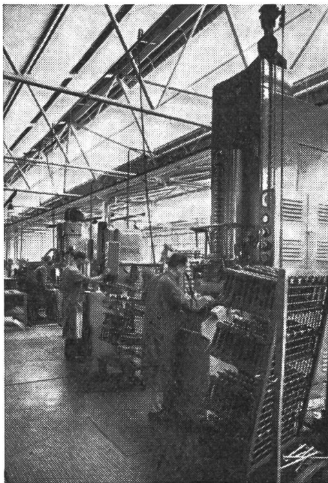
◀ Teilansicht Pleuelstangen-Fertigung
