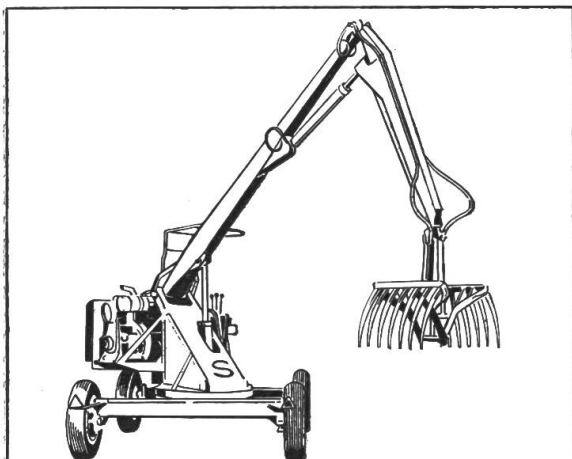
SEGALA der Mistladekran auf vier Rädern. Grosses Hubvermögen. Einfach in der Handhabung. Robuste Bauart.
