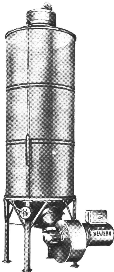
NEUERO-Silotrockner mit elektrischem Luftheitzer
