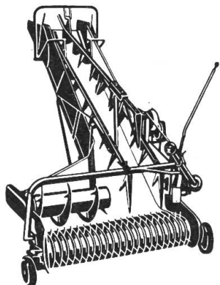
Kombi-Lader SL 160 mit Wurfband zum Laden von allen Futterarten wie Heu, Gras, Grünmais, Zuckerrübenlaub usw. Aufnahmebreite 1,6 m, Ladehöhe 3,3 m
