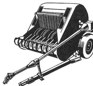
Niederdruck-Sammelpresse F 80 + F 81 zum Pressen und Laden von Heu und Stroh. Aufnahmebreite 1,4 m Stundenleistung 4 bis 8 Tonnen Jetzt mit Grünfutterelevators lieferbar
