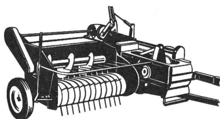
Hochdruck-Sammelpresse 214 B/D + C/B 300 für Heu und Stroh Aufnahmebreite 1,60 m, Stundenleistungen: Stroh 7 Tonnen, Heu 9 Tonnen
