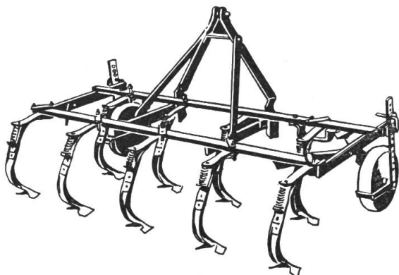
Kultivator mit 9 abgefederten Arnszinken mit Gänsefuss-Scharli.
