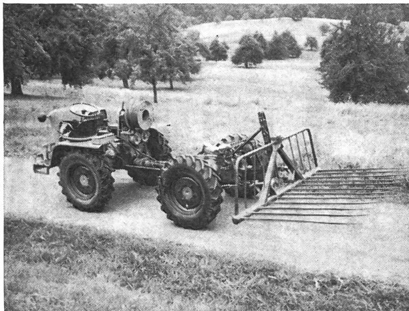
Abb. 1: Silo-Schwanz ohne Schutzlatte, aufgebaut am Merk-Pullax. Es dürfte jedermann einleuchten, dass die Spitzen im Strassenverkehr sehr gefährlich werden können,
