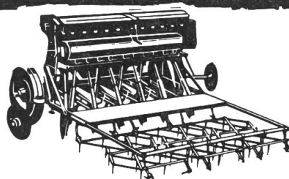
Hassia-Sämaschine
