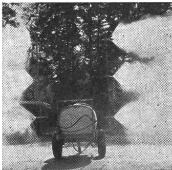
Bimoto-ARBOR-Zapfwellenwagen in Aktion Bimoto-TITAN-BH-III 75 l/min - 60 Atm. - 1000 Liter Holzfass - Pneus 9.00-13" - Podest - Schraubstütze - Vertikal-Spritzbarren für Hecken- und Busch-Anlagen
