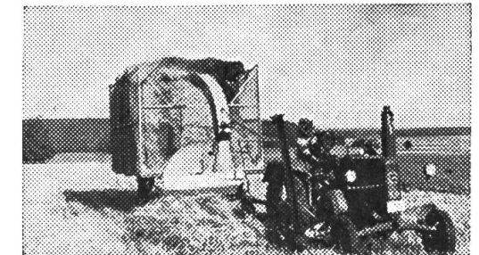
Krüger-Streuer als Häckselwagen
