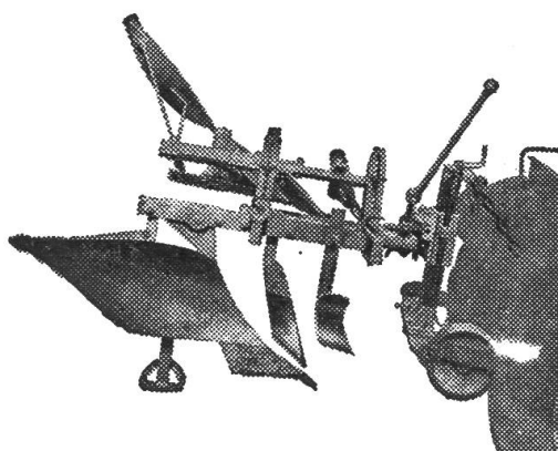
Winkeldrehpflug WD 60
