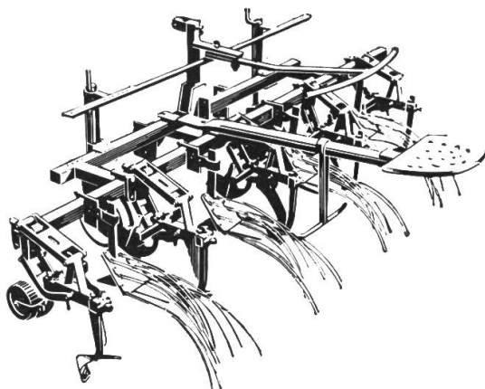
Vielfachgerät
