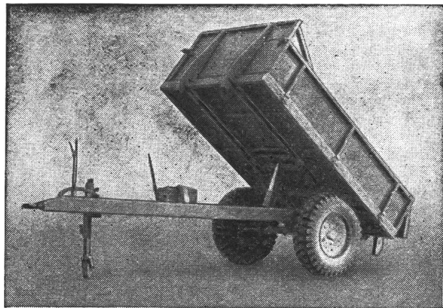
Universal-Anhänger als Kipper 1,5 m³ Inhalt, mit abgelegter Front- und Rückwand als Heu- und Graswagen verwendbar.
