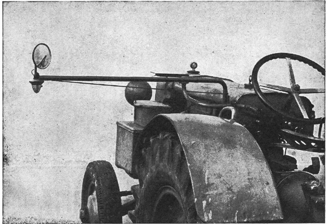
Ansicht von hinten des ausgeschwenkten Blink- und Spiegelgerätes «Argus».
