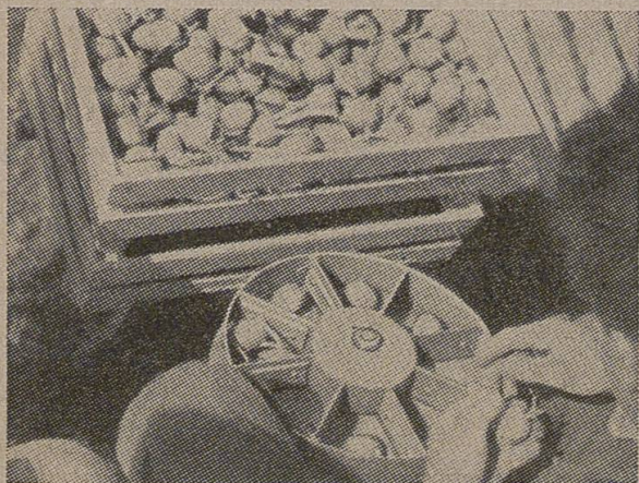
Patent-Setzautomat mit 8-teiligem Zellenrad beim Setzen von vorgekeimten Kartoffeln.
