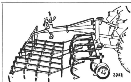
KOMBI-Kultivator/Egge
