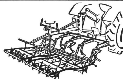
KOMBI-Kultivator/Rotorkrümler
