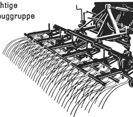
Abgefederte Gruppenwerkzeuge
