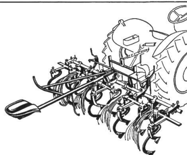
Traktoren-Vielfachgerät HARUWY
