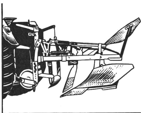
Winkeldrehpflug
