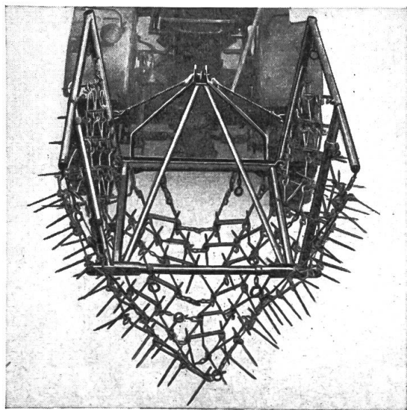
Netzegge, System Schönberger, dreiteilig, mit patentiertem Eggenträger, Seitenflügel hochgeklappt, in Transportstellung.
