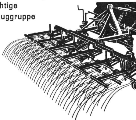
Abgefederte Gruppenwerkzeuge
