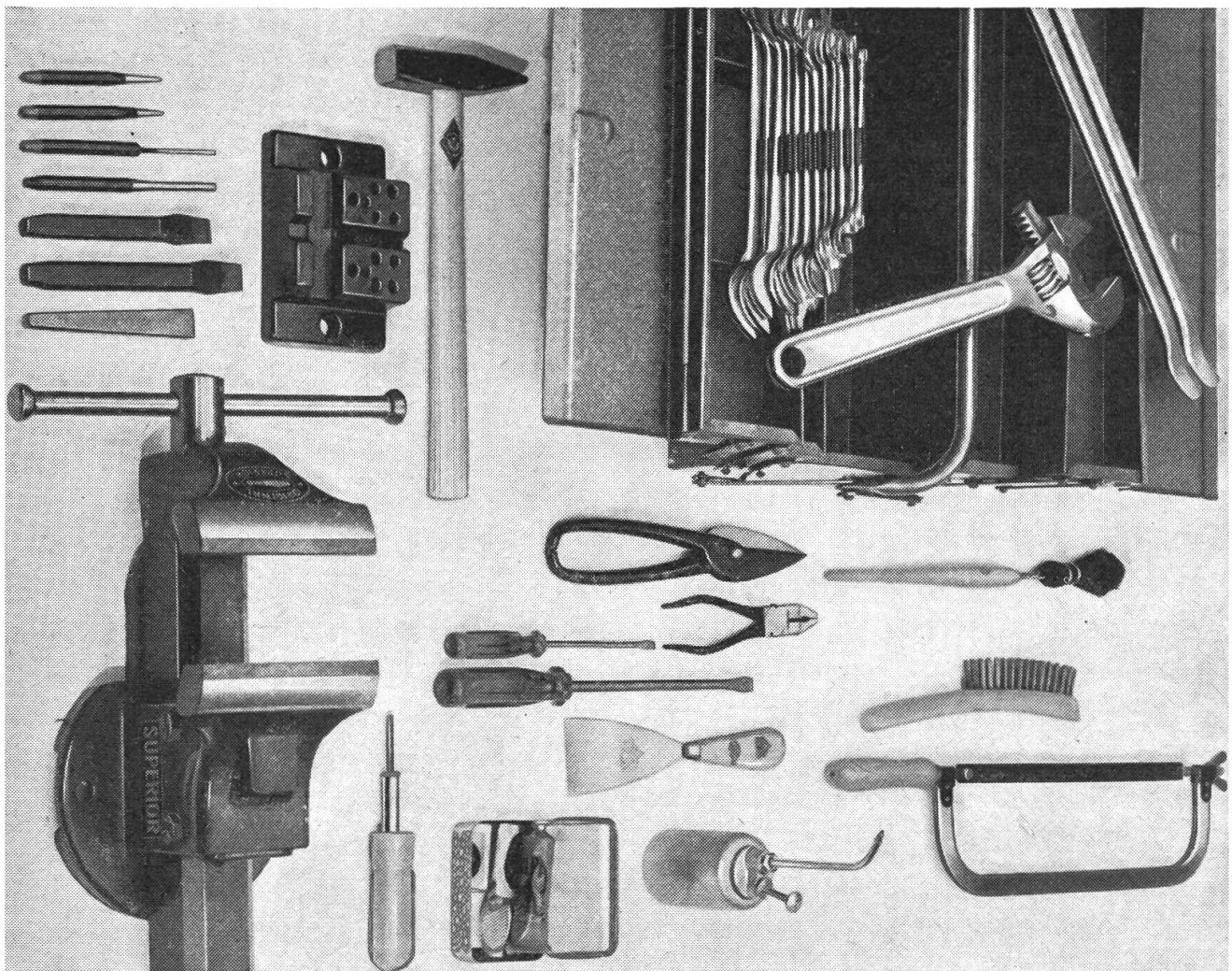
Abb. 1: Agro-Werkzeug-Basissatz
