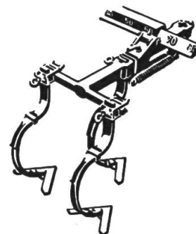
abgefederte Gruppenwerkzeuge
