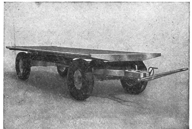
«WM»-Pneuwagen, 1,5—5 Tonnen Nutzlast, rostfreie Ganzmetallkonstruktion
