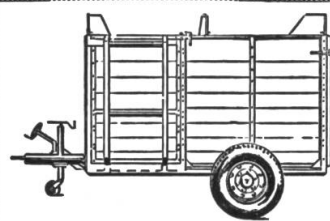
Viehwagen für Traktor oder Jeep
