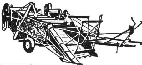
Type GM 4: Für Schlepperzug, mit Zapfwellenantrieb ab 25 PS, mit VW Aufbaumotor ab 12 PS Schlepper ausreichend, 1,60 m Schnittbreite, ca. 1500 kg Stundenleistung.
