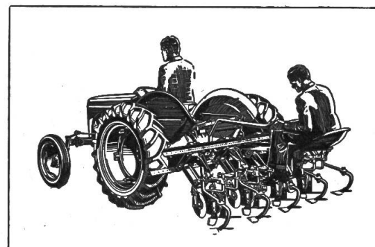
Hackgerät, steuerbar, leicht verstellbare Löffel- und Gänsefußscharen und Scheiben, Bedienung mit Feinsteuerern, 4-reihig (speziell für Zuckerrübenbau).
