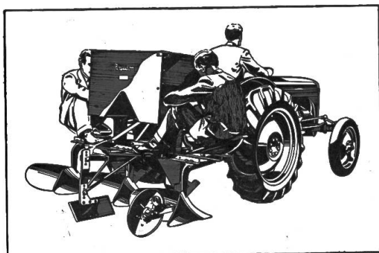
Kartoffelsetzmaschine, 2-reihig, 2-Mann-Bedienung (zum Aufbau auf Ferguson 3-Schar-Furchenzeiler). Saatgutbehälter für 175 kg Kartoffeln, ohne Behälter, für 6 Gitter keimendes Saatgut.
