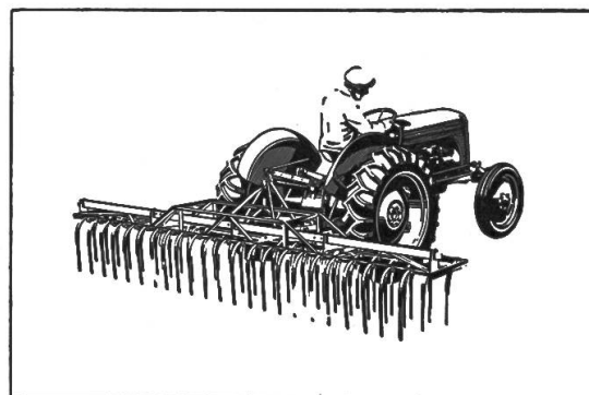
Unkrautstriegel für Saatfelder. Seitentelle aufklappbar (Transportstellung). — Arbeitsbreite 388 cm, Arbeitstiefe 6–10 cm.
