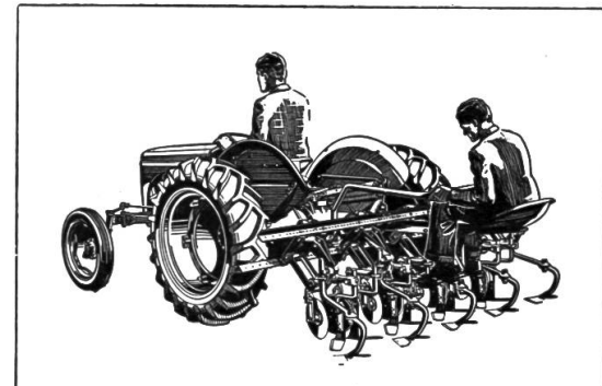
Hackgerät , steuerbar, leicht verstellbare Löffel- und Gänsefüßscharen und Scheiben, Bedienung mit Feinsteuermann, 4-reihig (speziell für Zuckerrübenbau).
