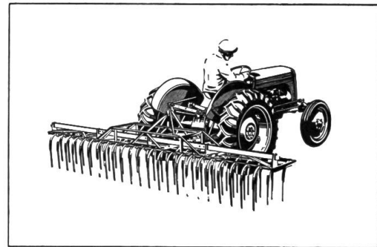
Unkrautstriegel für Saatfelder. Seitenteile aufklappbar (Transportstellung). — Arbeitsbreite 388 cm, Arbeitstiefe 6–10 cm.
