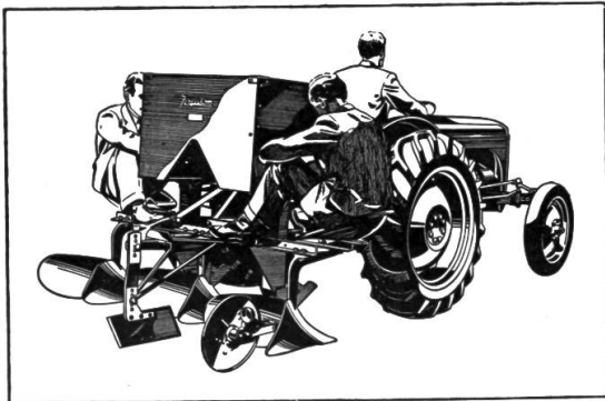
Kartoffelsetzmaschine , 2-reihig, 2-Mann-Bedienung (zum Aufbau auf Ferguson 3-Schar-Furchenzieher). Saatgutbehälter für 175 kg Kartoffeln, ohne Behälter, für 6 Gitter keimendes Saatgut.
