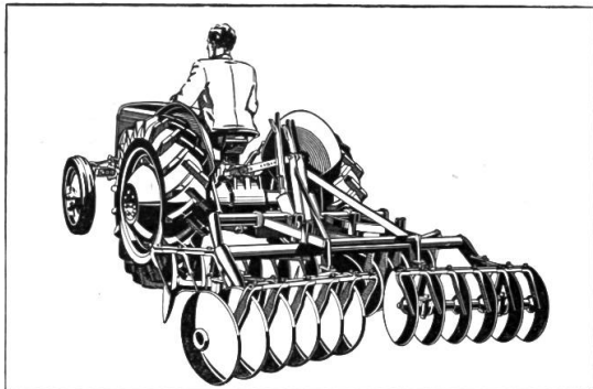
Getragene Scheibenegge , 3-Punkt-Aufhängung. 20 oder 24 Scheiben, 45 cm Durchmesser. Arbeitsbreiten 180–210 cm. Äusserst solide, leistungsfähige Konstruktion.
