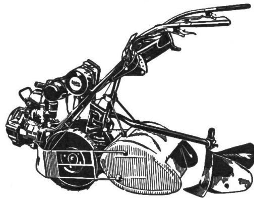
AGRIA-Universal 5 PS 200 ccm als Bodenfräse mit Häufler u. Blattabweiser.
