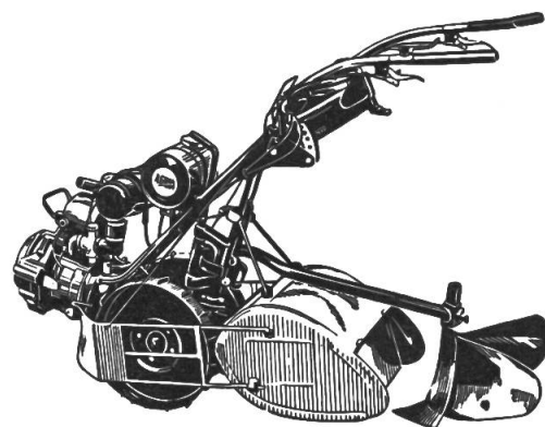
AGRIA-Universal 5 PS 200 ccm als Bodenfräse mit Häufner u. Blattabweiser. Kompl. Bodenfräse ab Fr. 1526.—.
