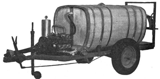
Royal-Hochdruck-Spritze für Zapfwellenantrieb
