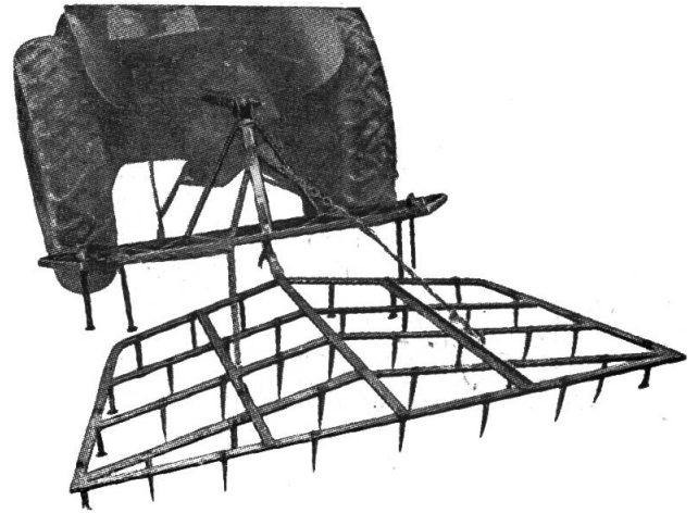
Erismann-Ackeregge an Dreipunktanbaurahmen
