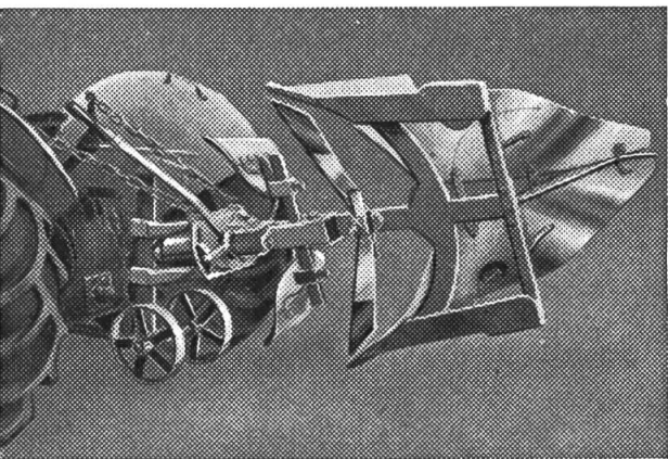
Henriod, mit Stützrädern
