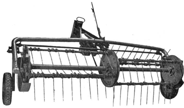
Graszettmaschine Wängi
