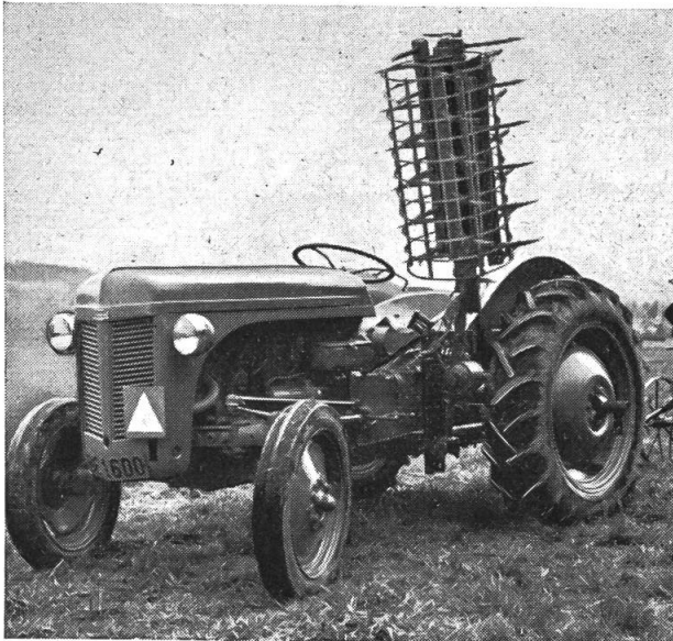
Sonnaillon-Anbauegge (seitlich)
