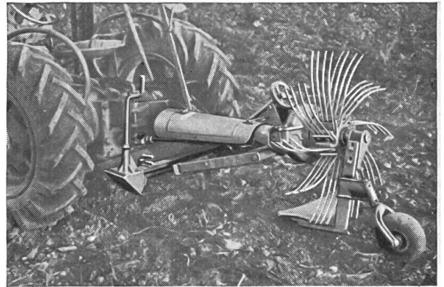
Kartoffelgraber Schmotzer
