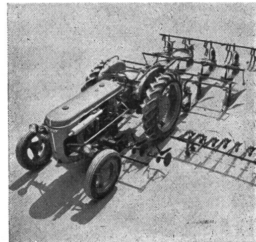
Vevey Hackgeräte
