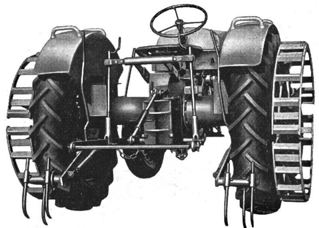
Meili-Gitterräder und -Spurlockerer
