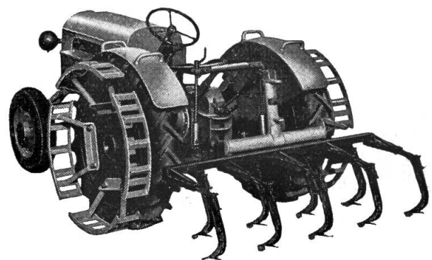
Meili-Gitterräder und Kultivator
