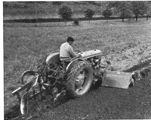
Vevey-Anbauegge (seitlich)
