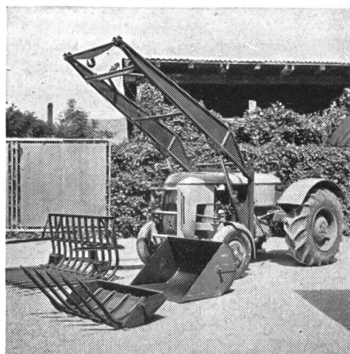
Frontlader Wittenburg-Vevey
