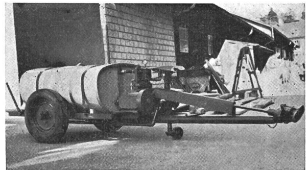
Royal-Hochdruck-Spritze für Zapfwellenantrieb
