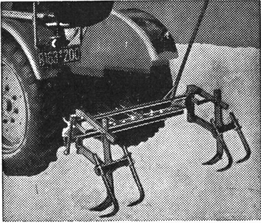
Degenhart-Spurlockerer (Griesser, Andelfingen)
