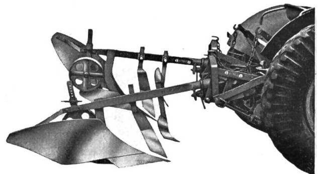
Althaus «Dominus» (Wechselpflug)
