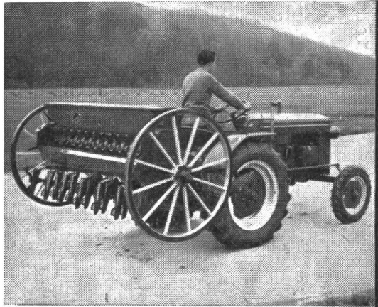
Anbau-Sämaschine mit Feinsäpparat
