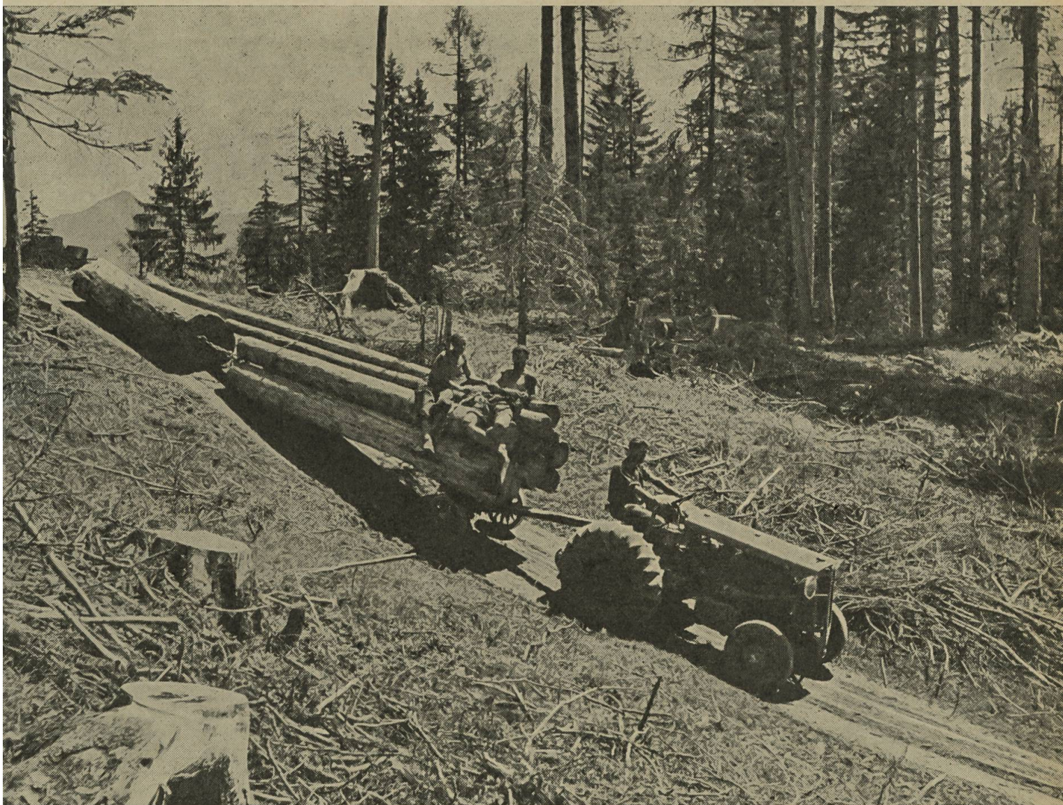
Hürlimann Diesel beim Holztransport im Gebirge
