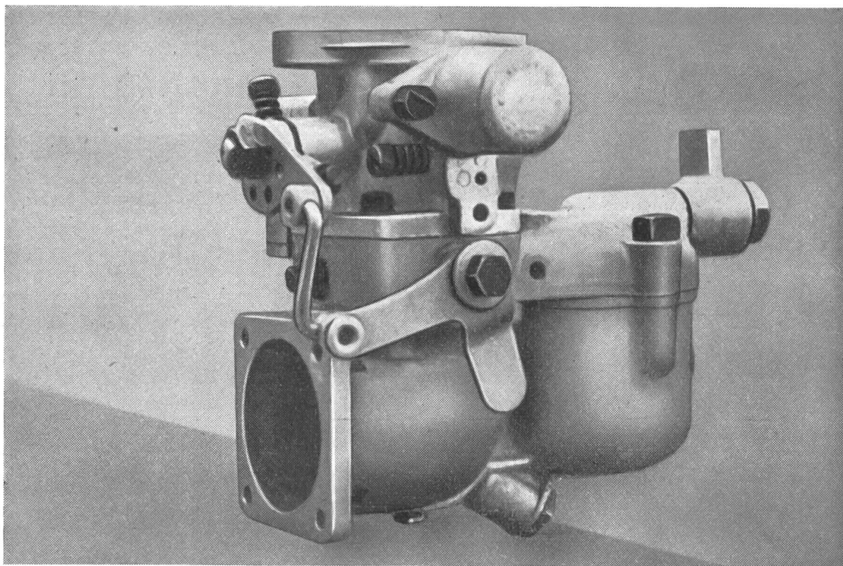
Fig. 1: Solex Steigstromvergaser neuerer Ausführung.
