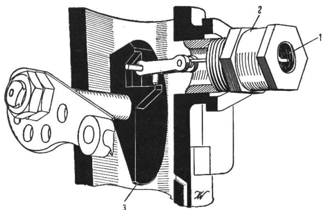
Fig. 7: Drehzahlbegrenzer.
