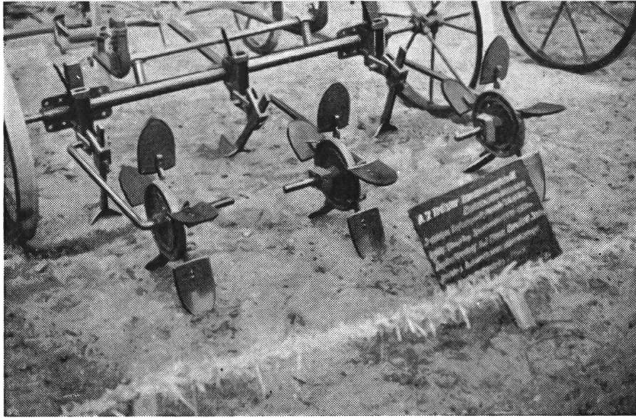
Lehrschau «Kartoffelkulturgerät»
