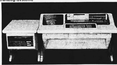
RUF-Computer mit Plattenspeichern, mit Floppy-Disketten, mit oder ohne Magnetkonten
